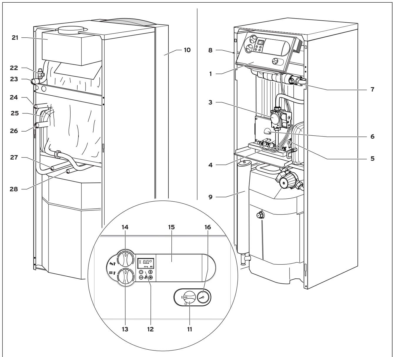
Fig. 1.2 Relación de los elementos funcionales
