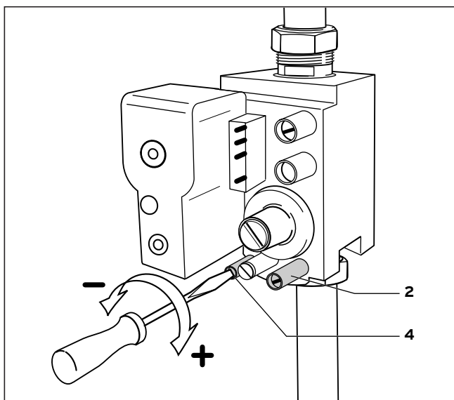
Fig. 5.2 Regulación de la presión de la boquilla
