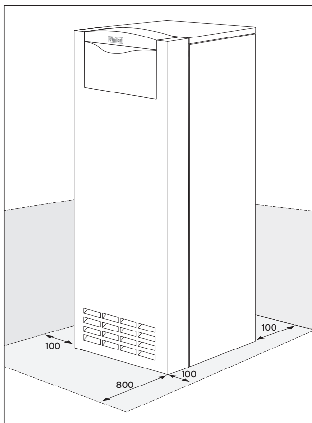
Fig. 3.2 Distancias mínimas
