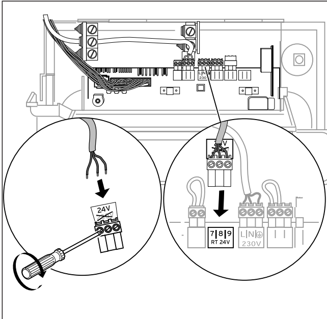
Fig. 4.6 Conectar el regulador a 7-8-9
