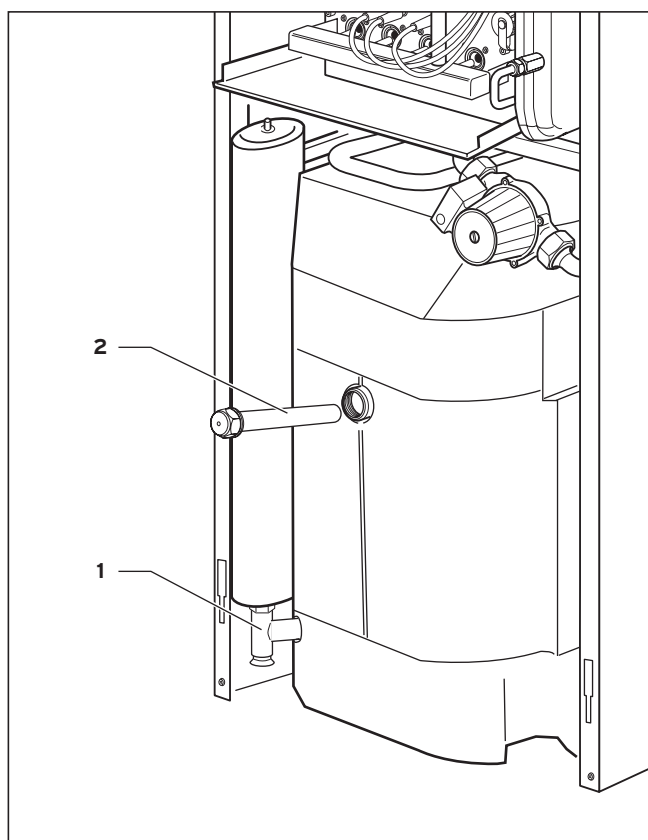
Fig. 7.5 Manutenzione dell'anodo di protezione
