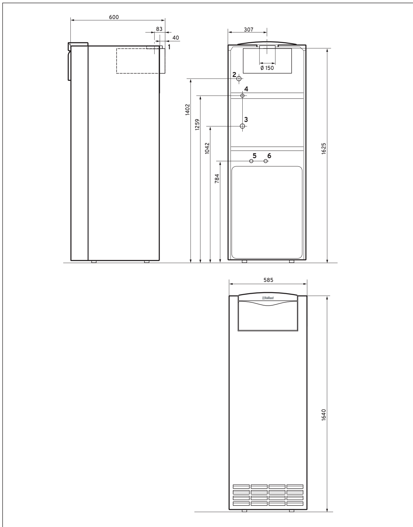
Fig. 3.1 Dimensiones VKC
