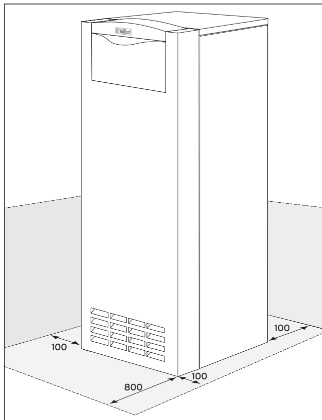
Fig. 3.1 Distanze minime
