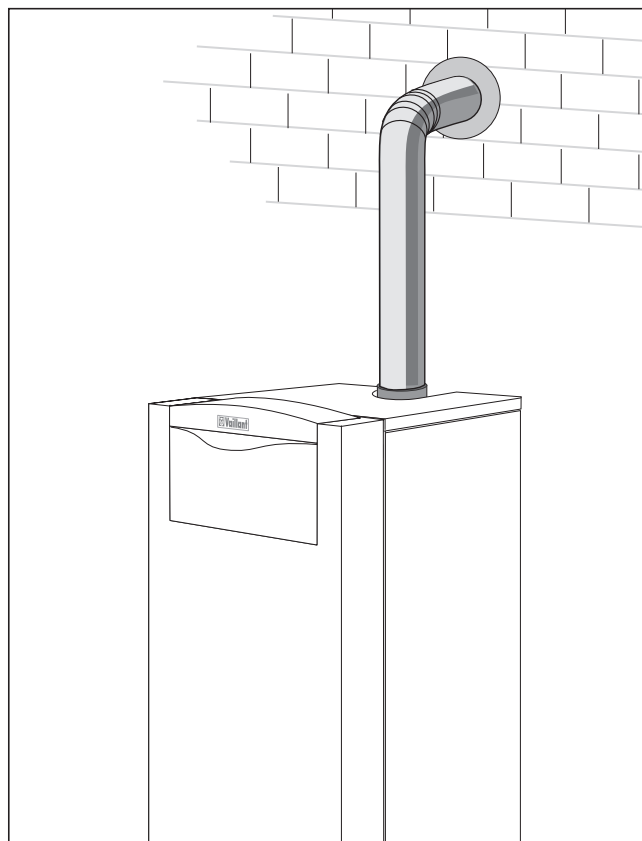
Fig. 4.3 Montaje del tubo salida de gases
