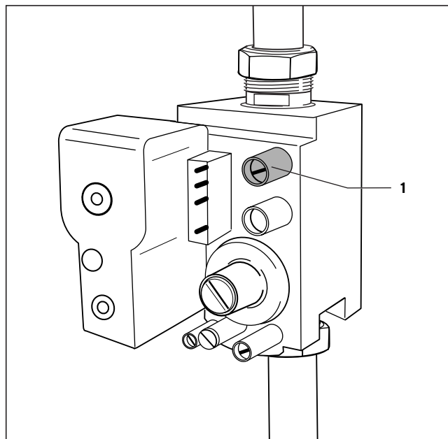
Fig. 5.1 Presión de conexión tubo de medición
