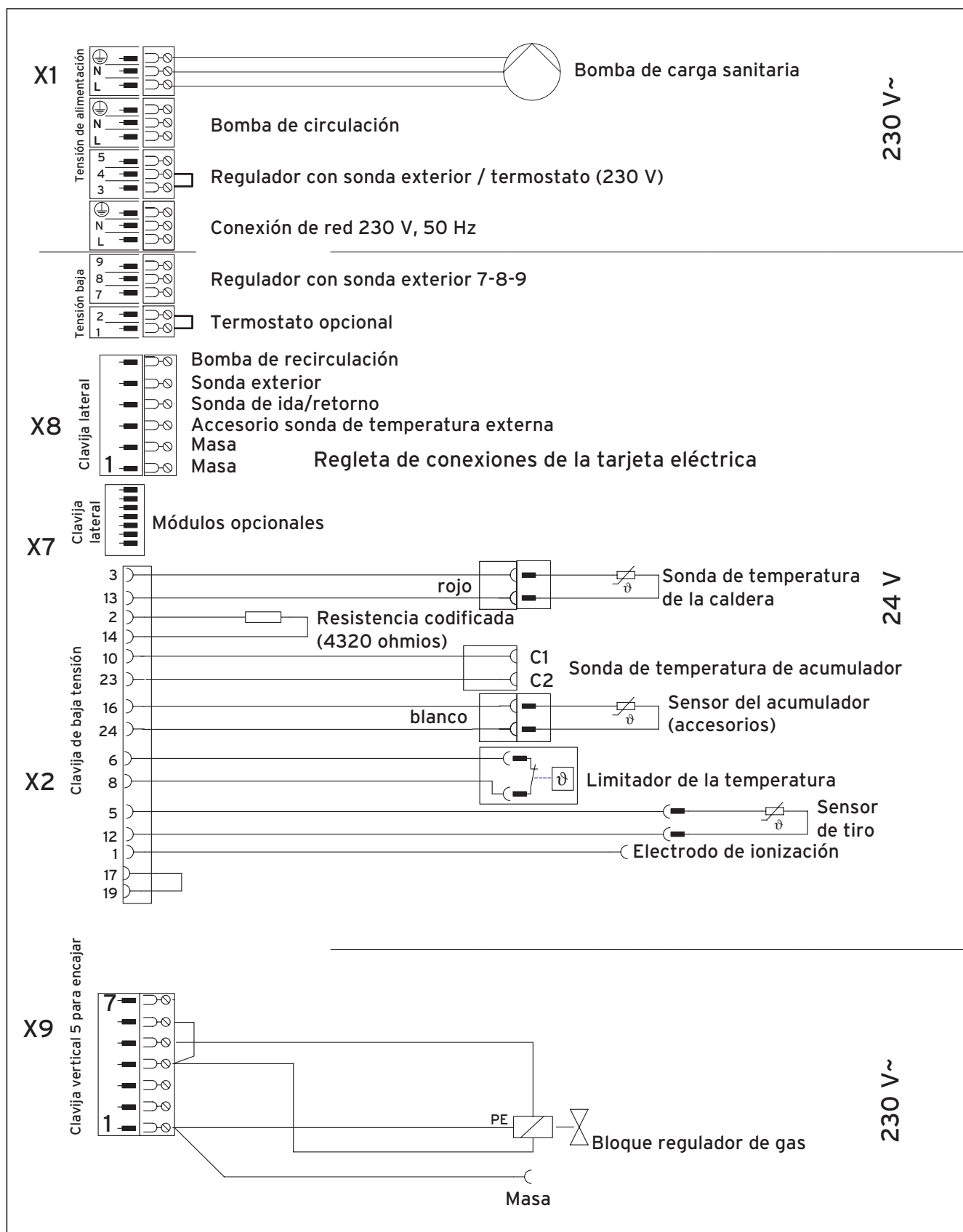
Fig. 4.5 Conexiones eléctricas atmoVIT combi
