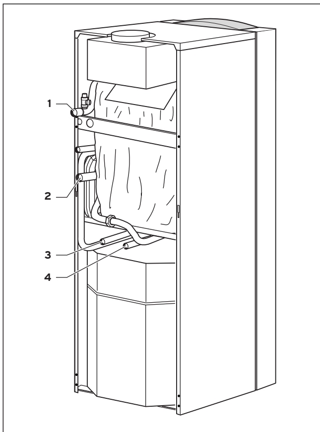
Fig. 4.1 Conexión en el lado de la calefacción
