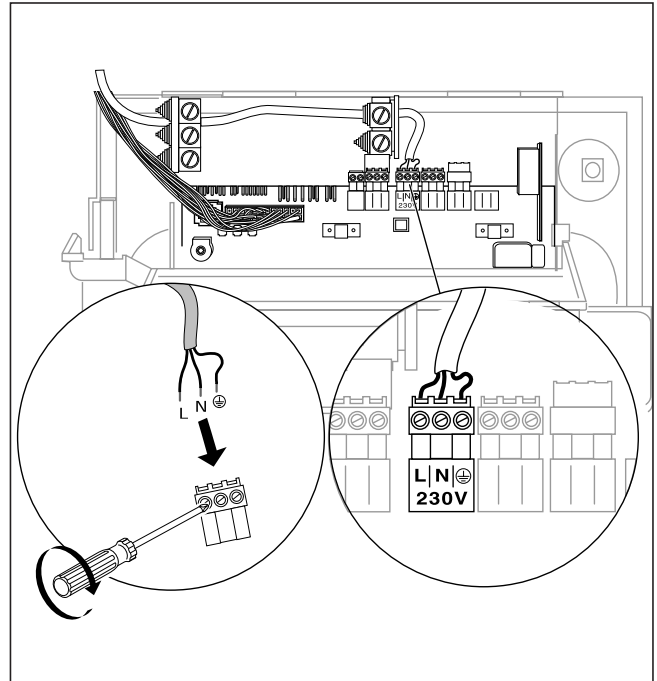
Fig. 4.4 Conectar la alimentación desde la red
