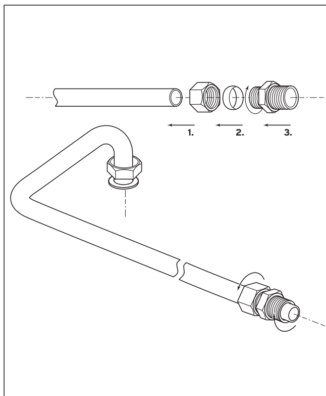
Fig. 4.2 Conexión de gas
