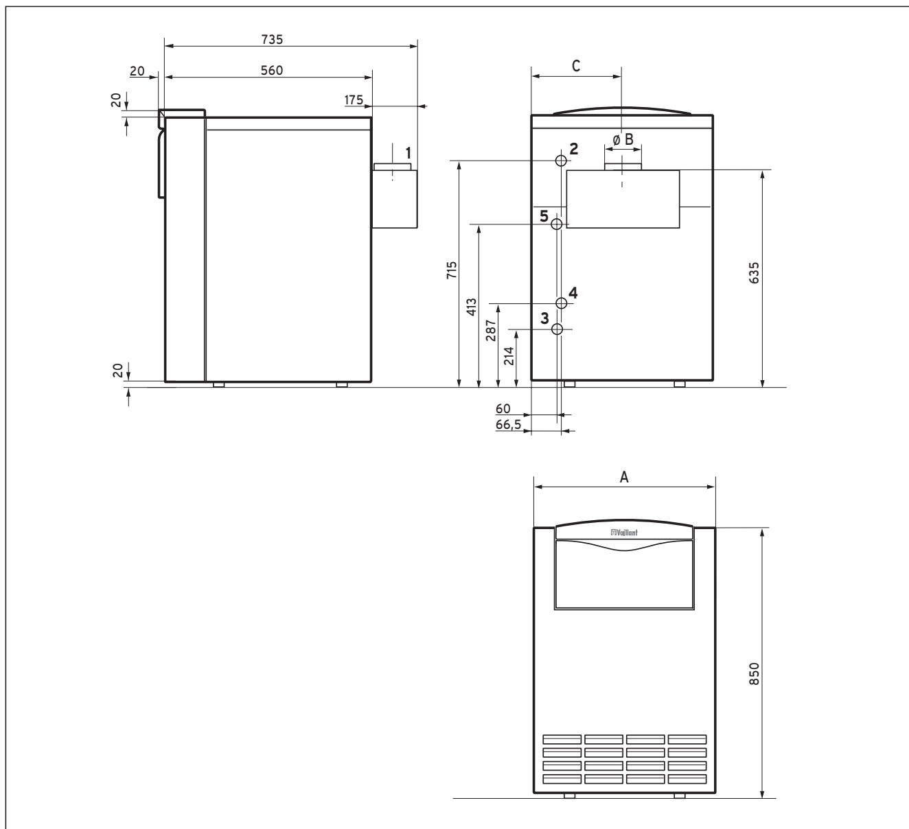
Fig. 3.3 Dimensioni dei modelli VK
