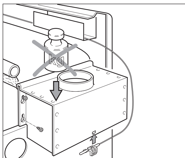
Fig. 3.2 Montaggio della cappa antivento
