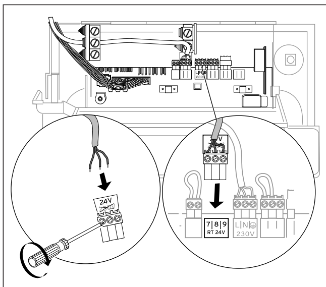
Fig. 4.7 Collegamento termostato modulante o VRC 7-8-9
