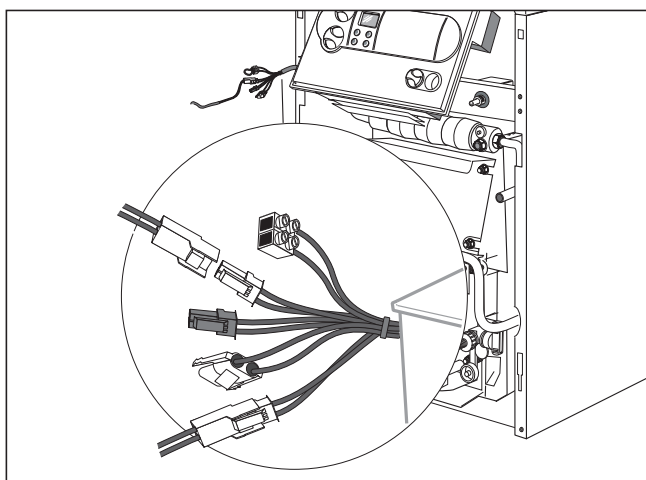
Fig. 4.6 Collegamento delle sonde
