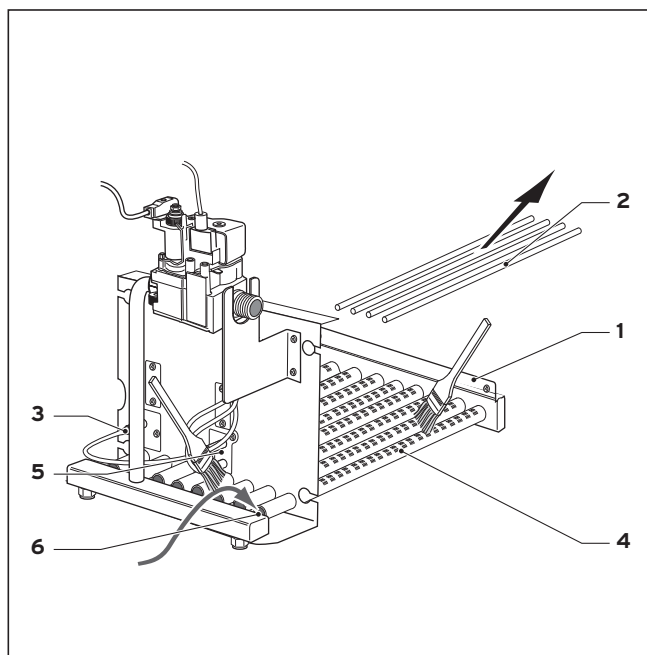
Fig. 7.3 Pulizia del bruciatore
