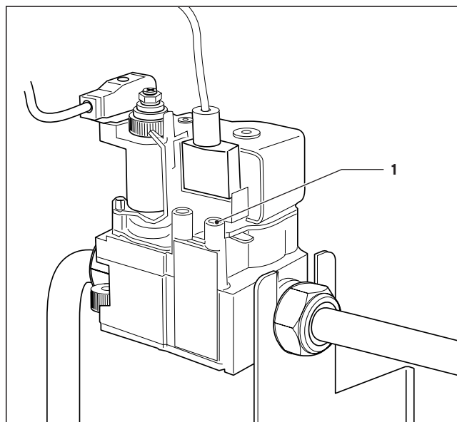
Fig. 5.1 Raccordo per la misurazione della pressione di allacciamento
