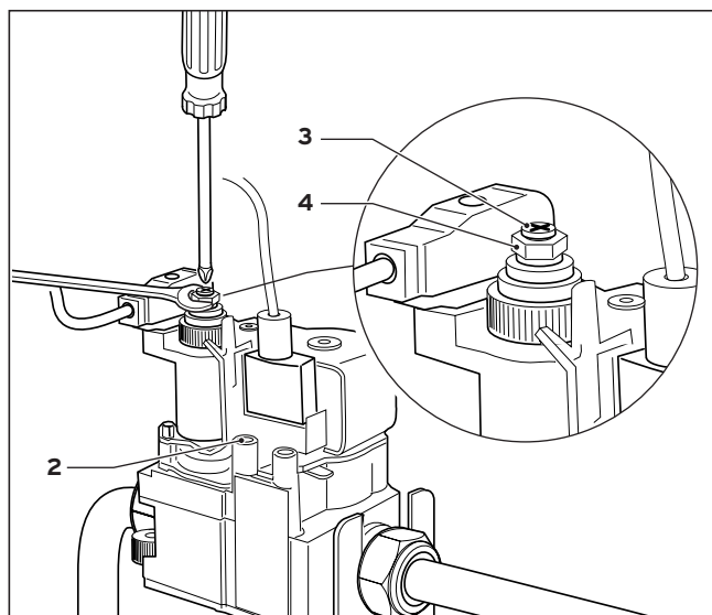
Fig. 5.2 Montaggio dell'ugello del gas
