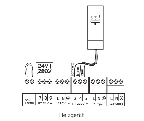
Abb. 10.1 Elektrischer Anschluss
