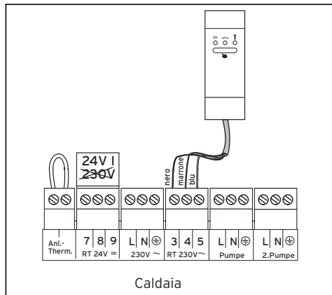
Fig. 10.1 Allacciamento elettrico
