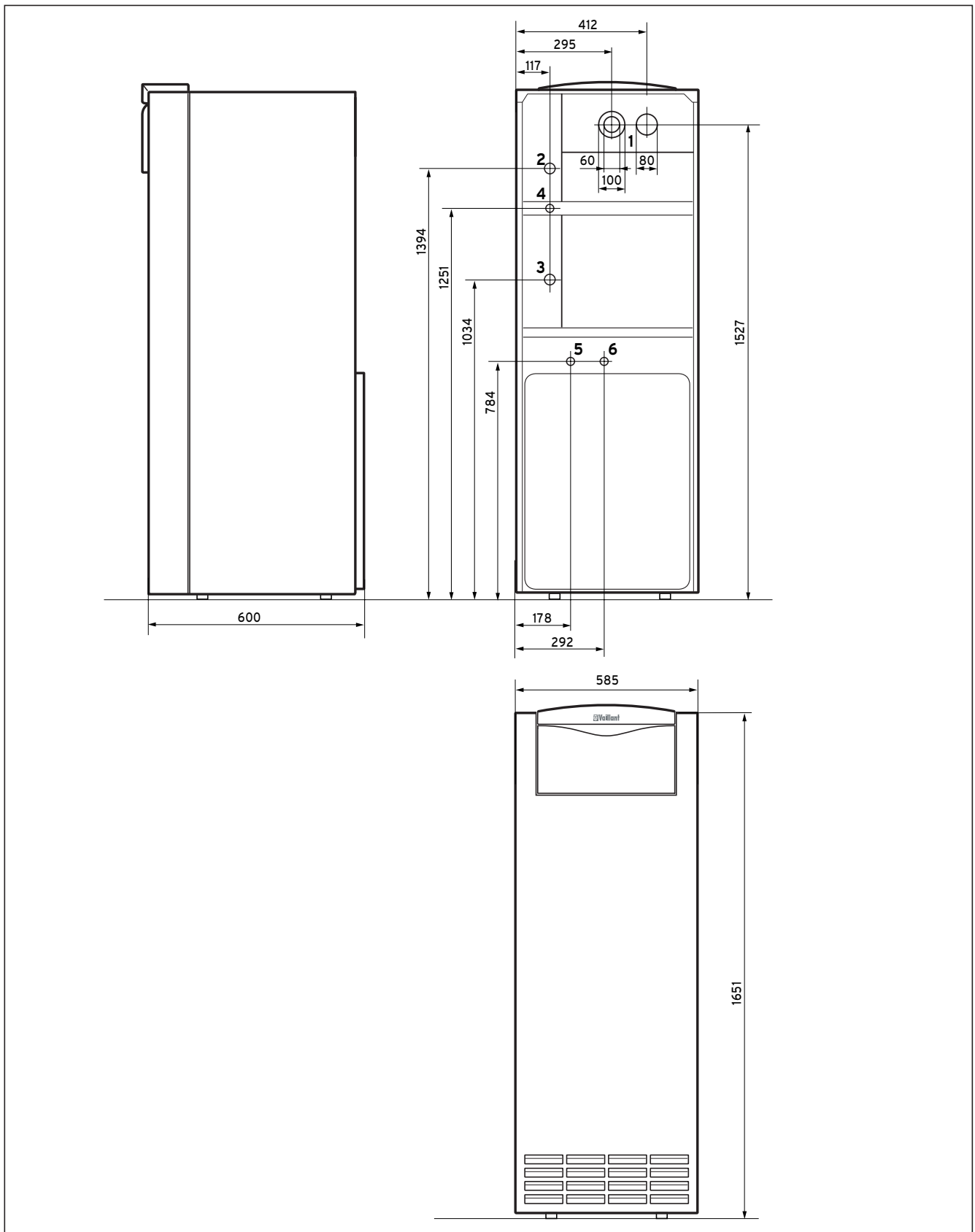
Fig. 3.1 Dimensiones VKC
