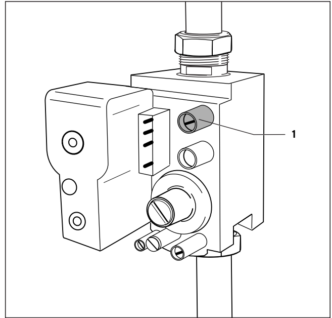
Fig. 5.1 Presión de conexión tubo de medición
