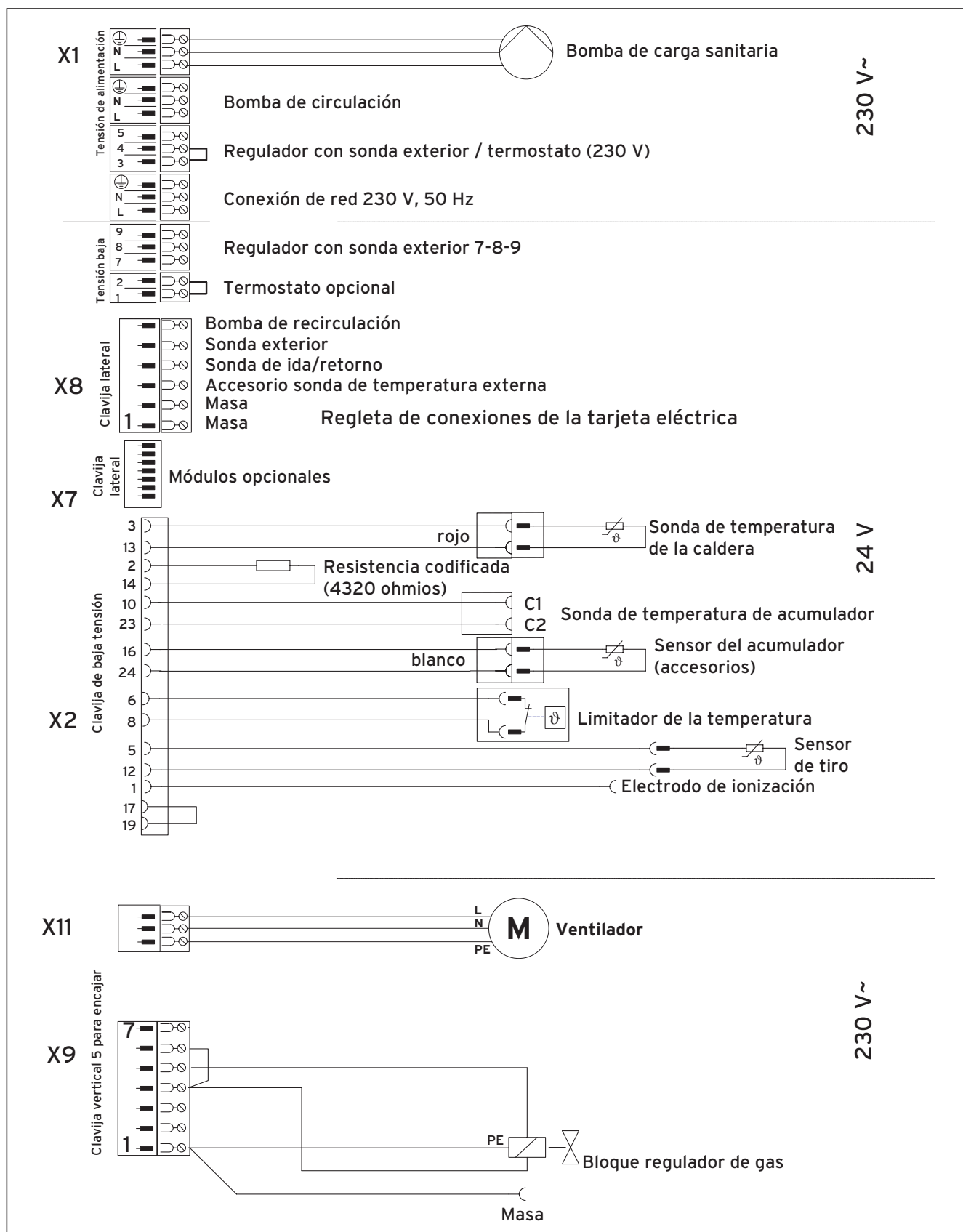
Fig. 4.5 Conexiones eléctricas turboVIT combi
