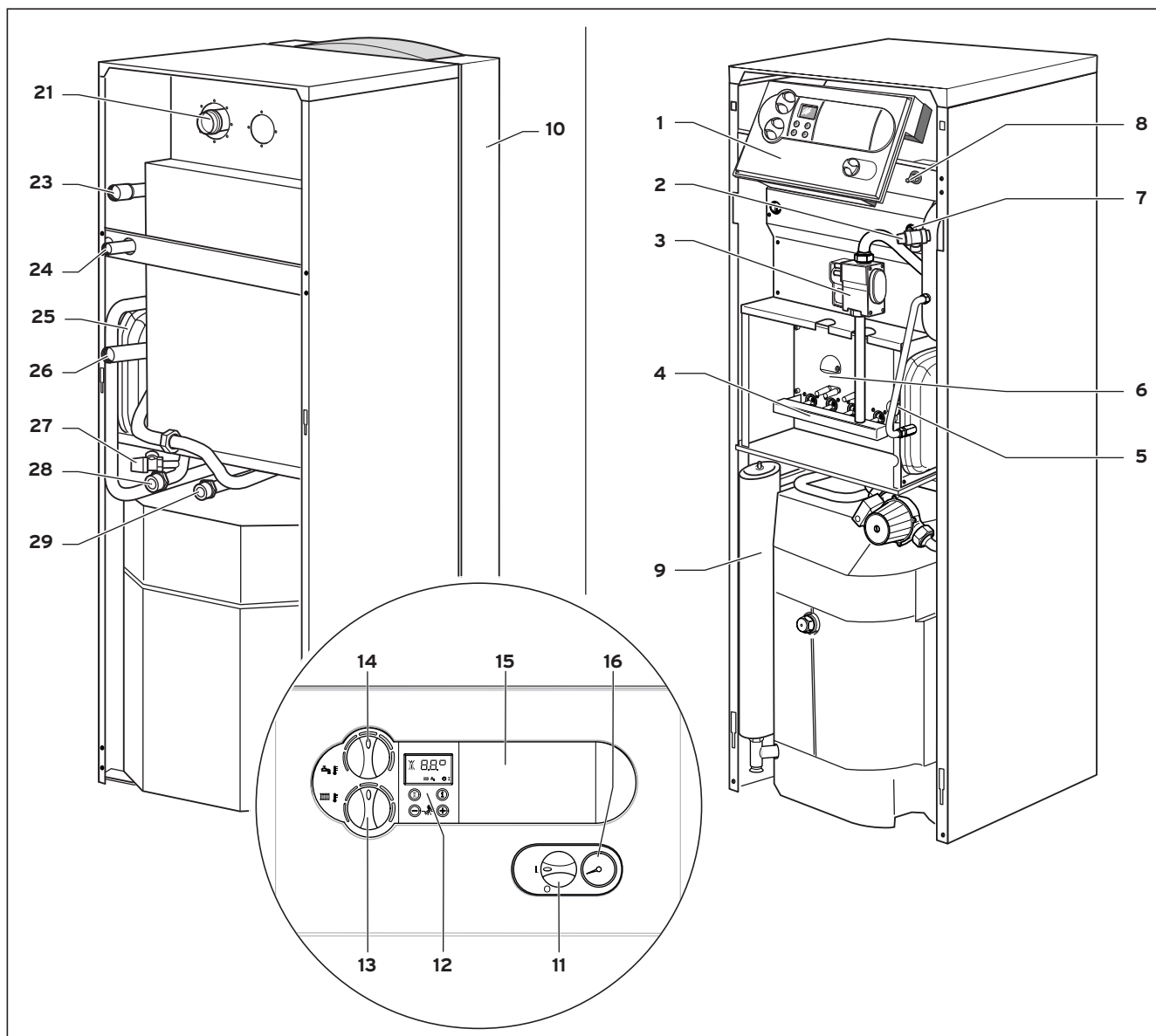
Fig. 1.2 Relación de los elementos funcionales
