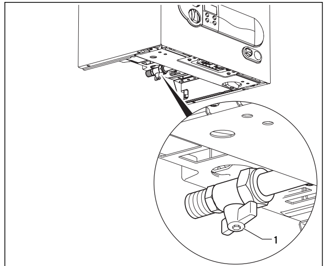
Fig. 5.1 Raccordo del gas
