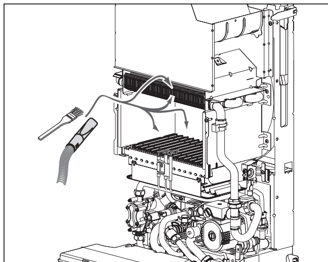
Fig. 8.1 Pulizia del bruciatore e dello scambiatore termico primario senza smontare (poca sporcizia)
