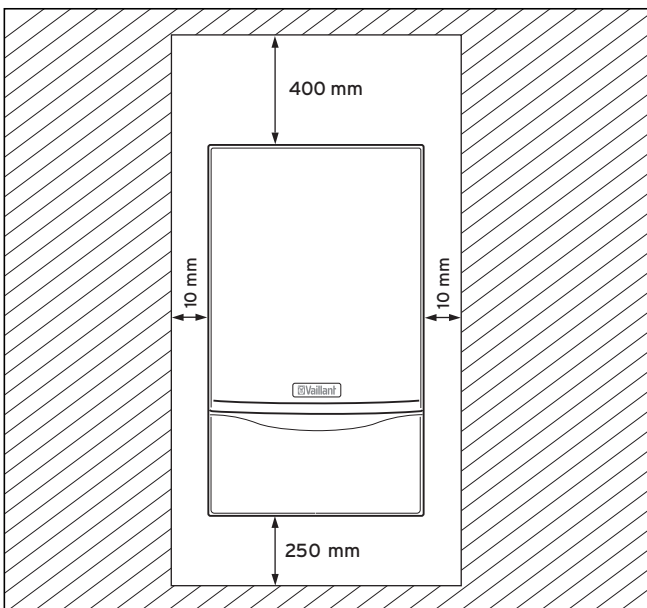
Fig. 4.3 Distanze minime richieste/spazio per il montaggio
