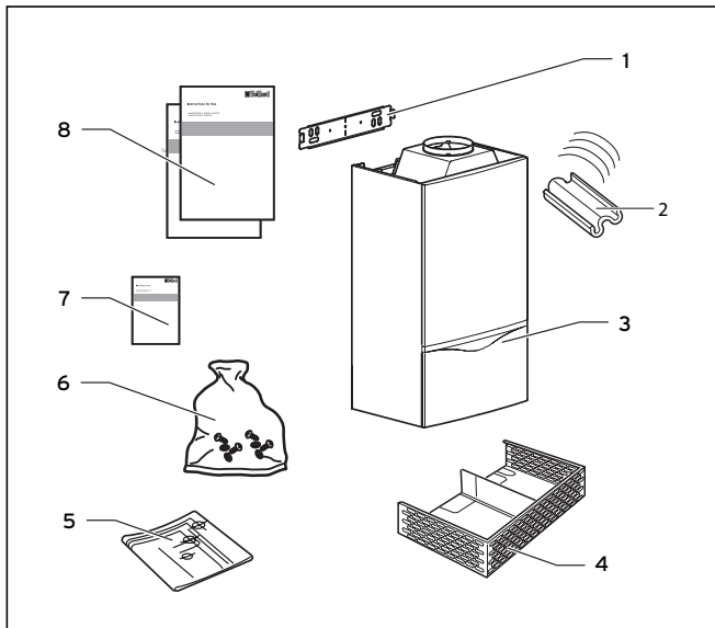
Fig. 4.1 Dotazione
