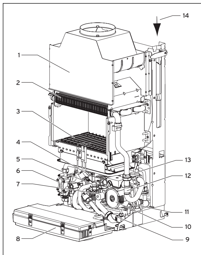
Fig. 2.1 Elementi funzionali
