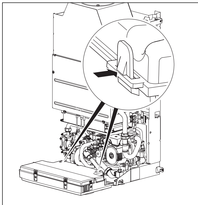
Fig. 5.6 Apertura del pannello posteriore del pannello di controllo
