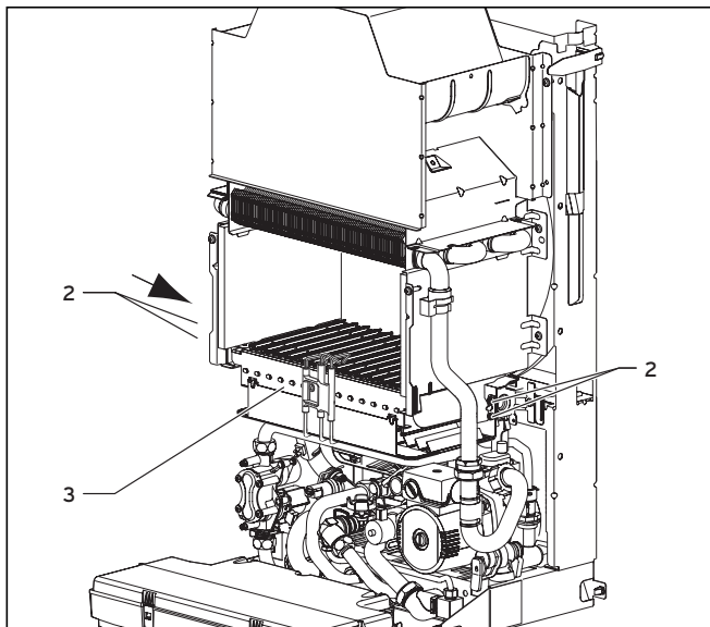
Fig. 8.3 Pulizia dello bruciatore smontandolo (sporcizia tenace)
