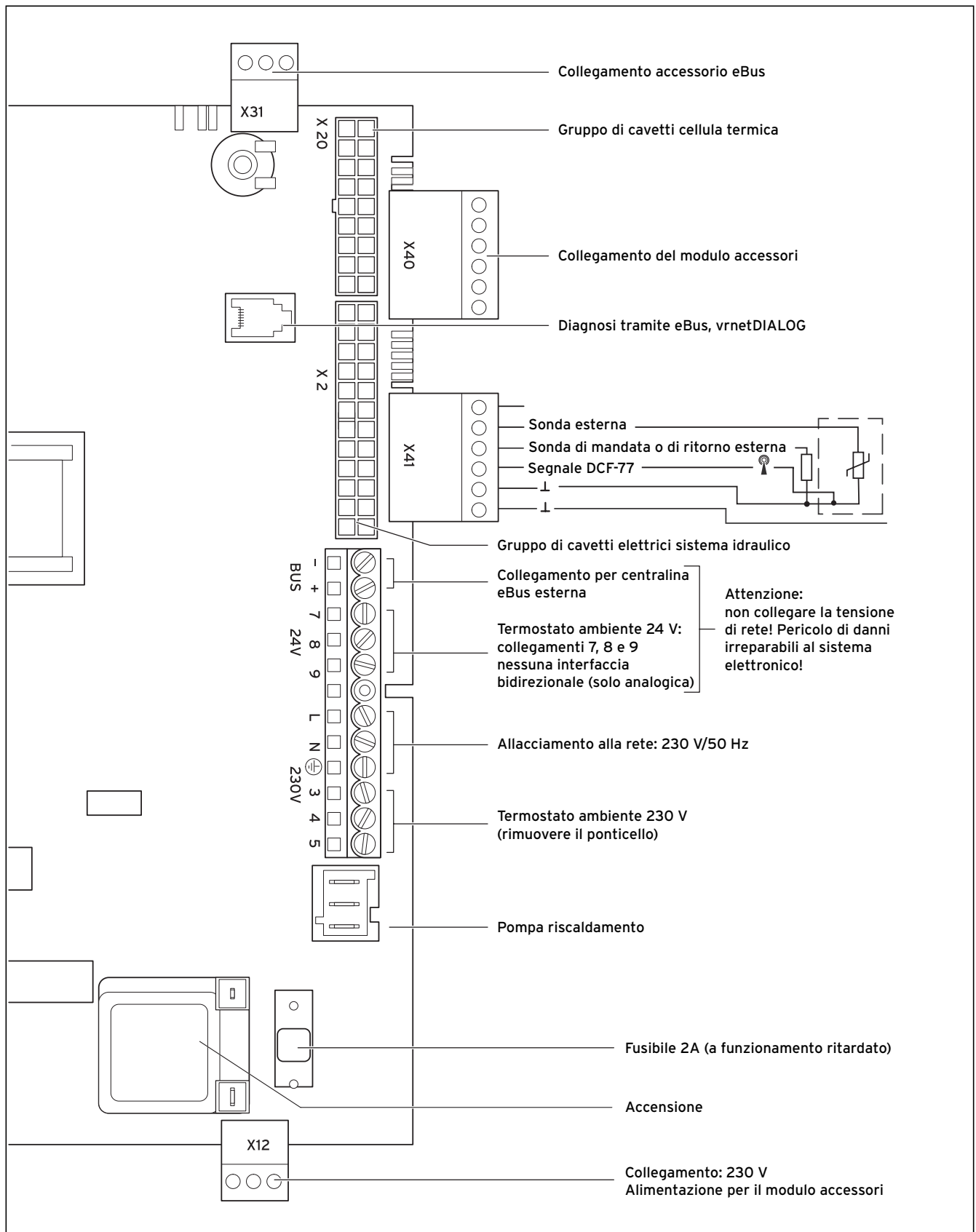
Fig. 5.8 Schema degli allacciamenti atmoBLOCK pro Balkon
