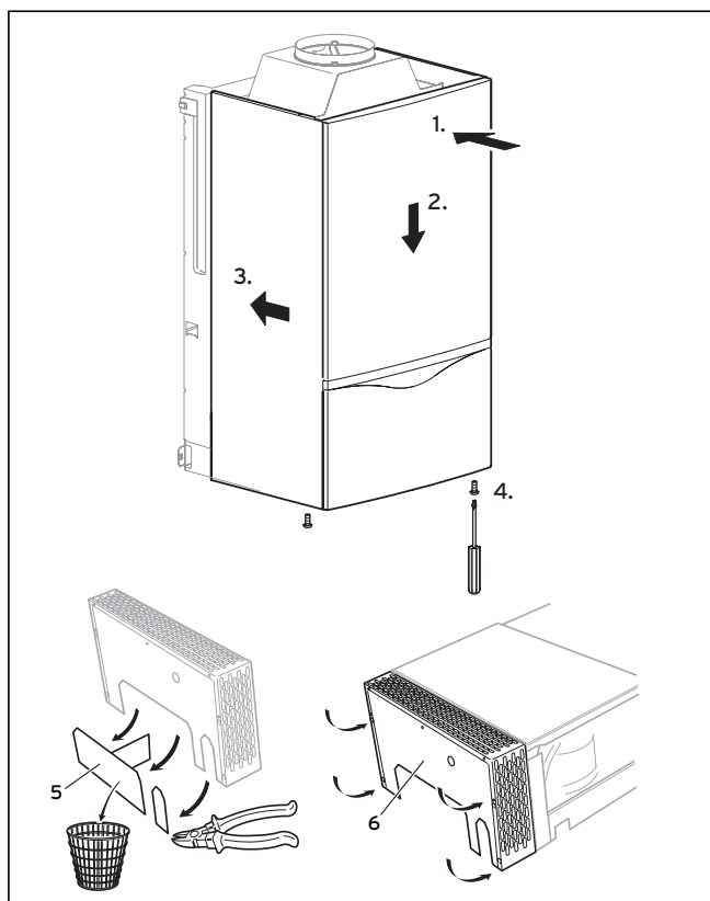
Fig. 4.7 Montaggio della copertura della caldaia
