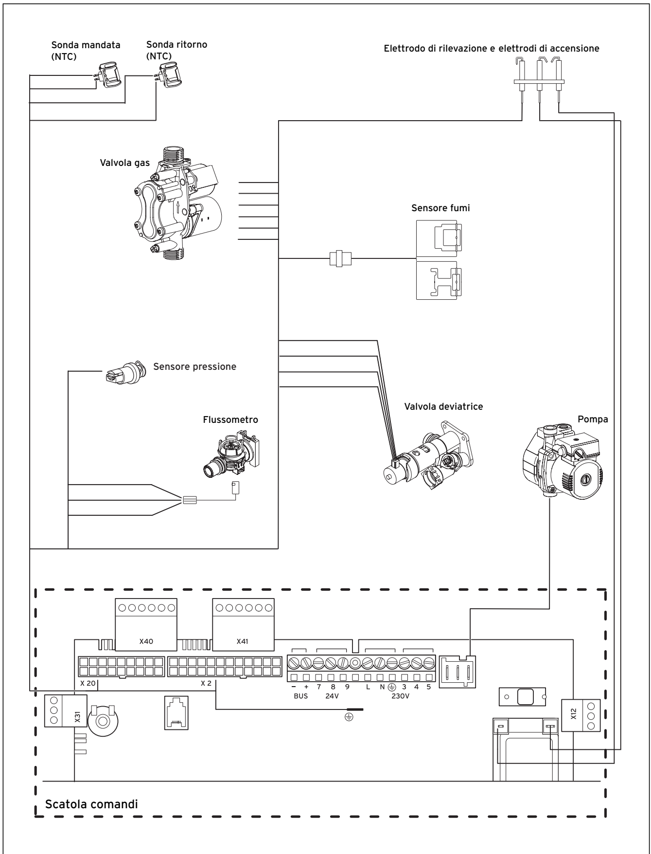
Fig. 5.9 Schema di cablaggio atmoBLOCK pro Balkon
